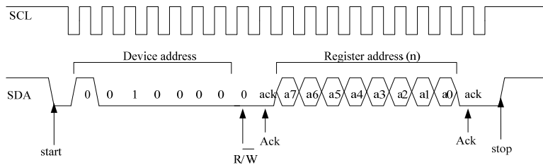
Step1: 配置寄存器地址 (写操作)
