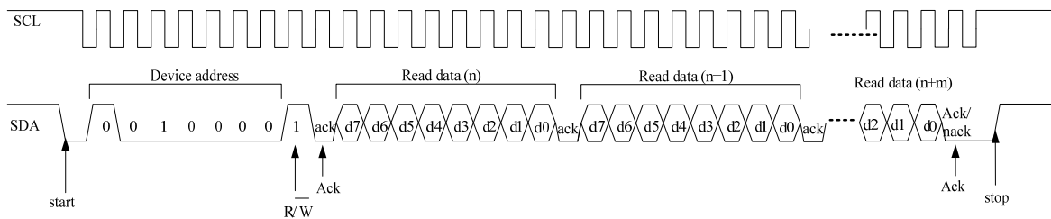
Step2: 读寄存器值 (i2c 连续读操作)
